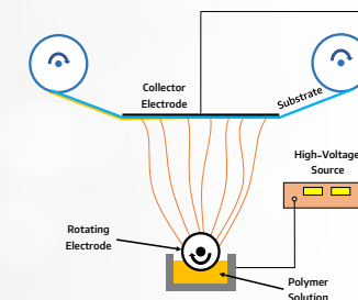
无针电纺
