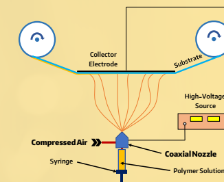
喷吹式电纺
